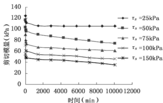
图 5 \sigma=100\text{kPa} , \omega=16.2\% 时剪切模量时间曲线
